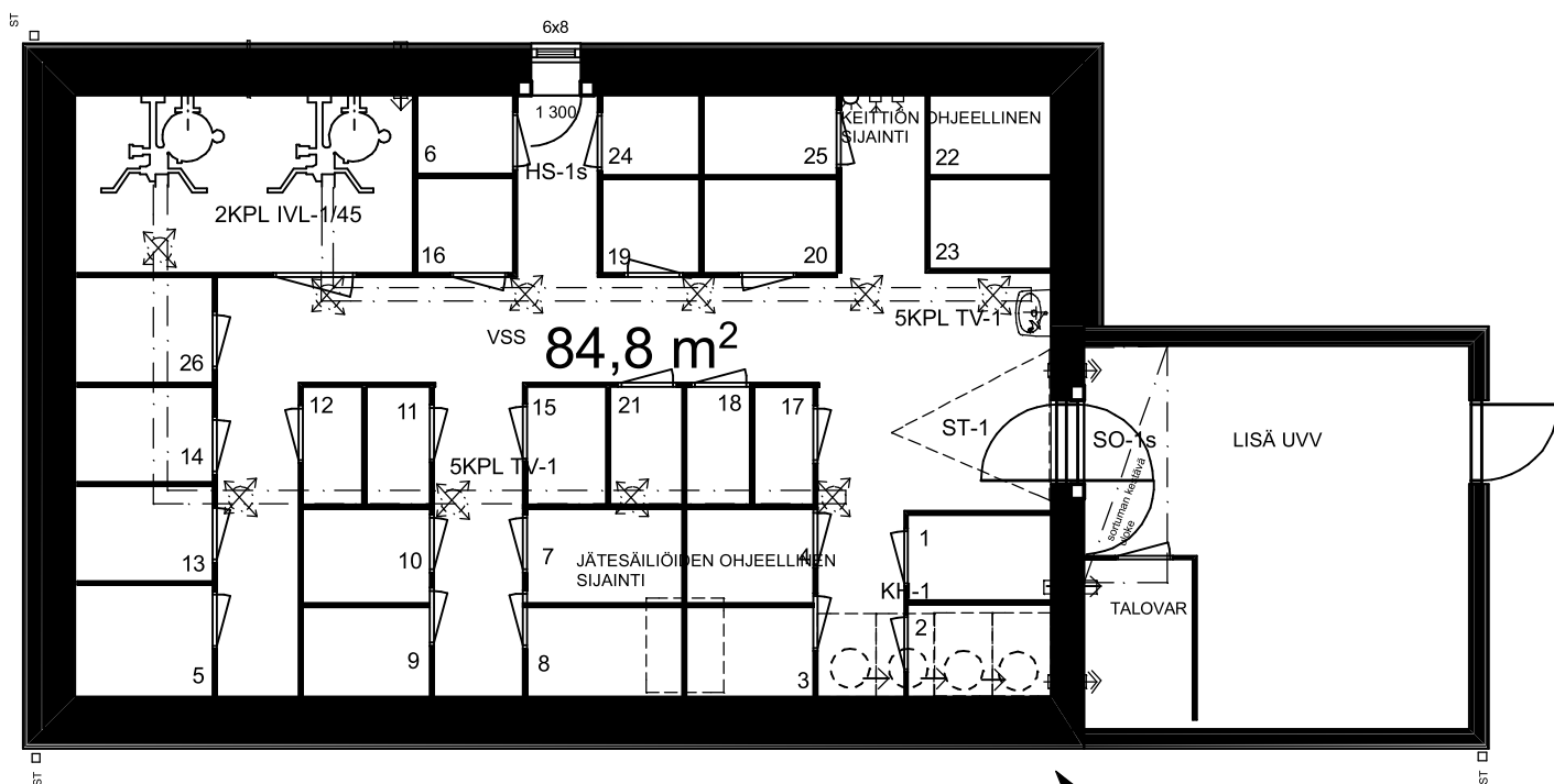
POHJAPIIRROS 1. KERROS, VSS / IRTVAR
